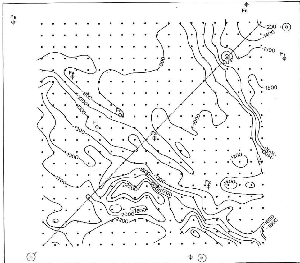
Fig. 12. Basement map. (a) Depth below sea level; (b) cross-section; (c) wells. [Carte en courbes de niveau du socle. (a) Profondeurs sous le niveau de la mer; (b) coupe d'interprétation; (c) forages.]
